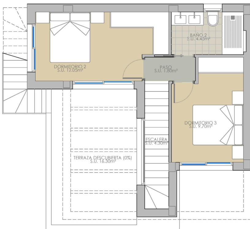
PLANTA PISO OPCIÓN 1
