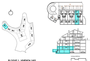
BLOQUE 1 - VIVIENDA 1402
