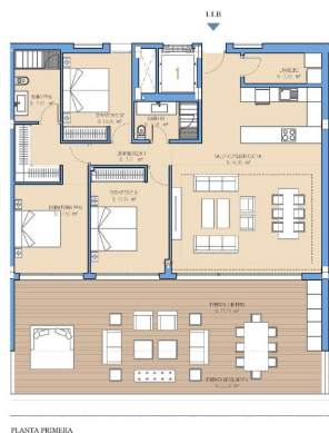
PLANTA PRIMERA
