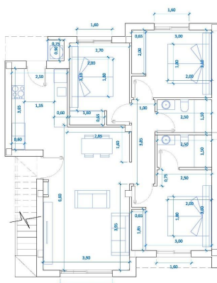
PLANTA MODELO A
