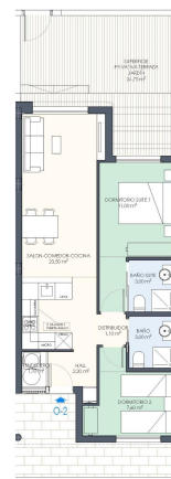
BLOQUE OESTE - PLANTA BAJA : VIVIENDA O-2
