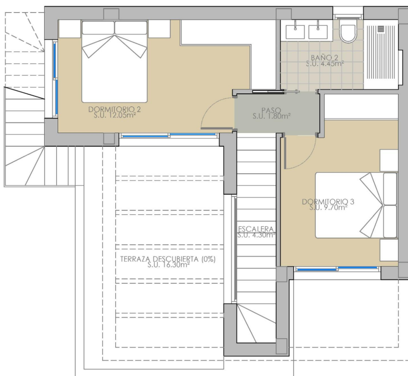
PLANTA PISO OPCION 1
